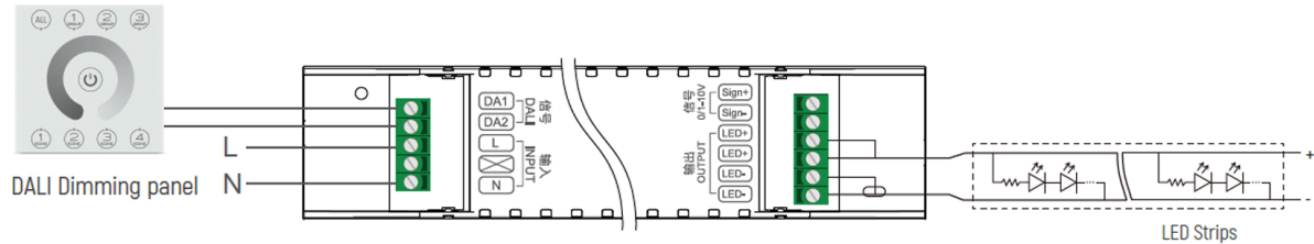
DALI Wiring
