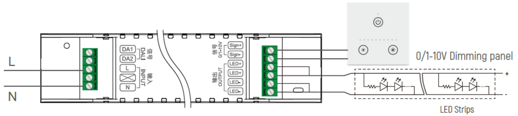
0/1-10V Wiring
